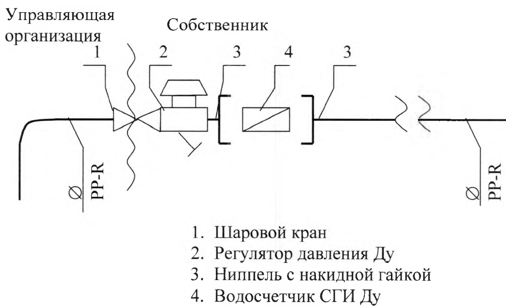
Схема
